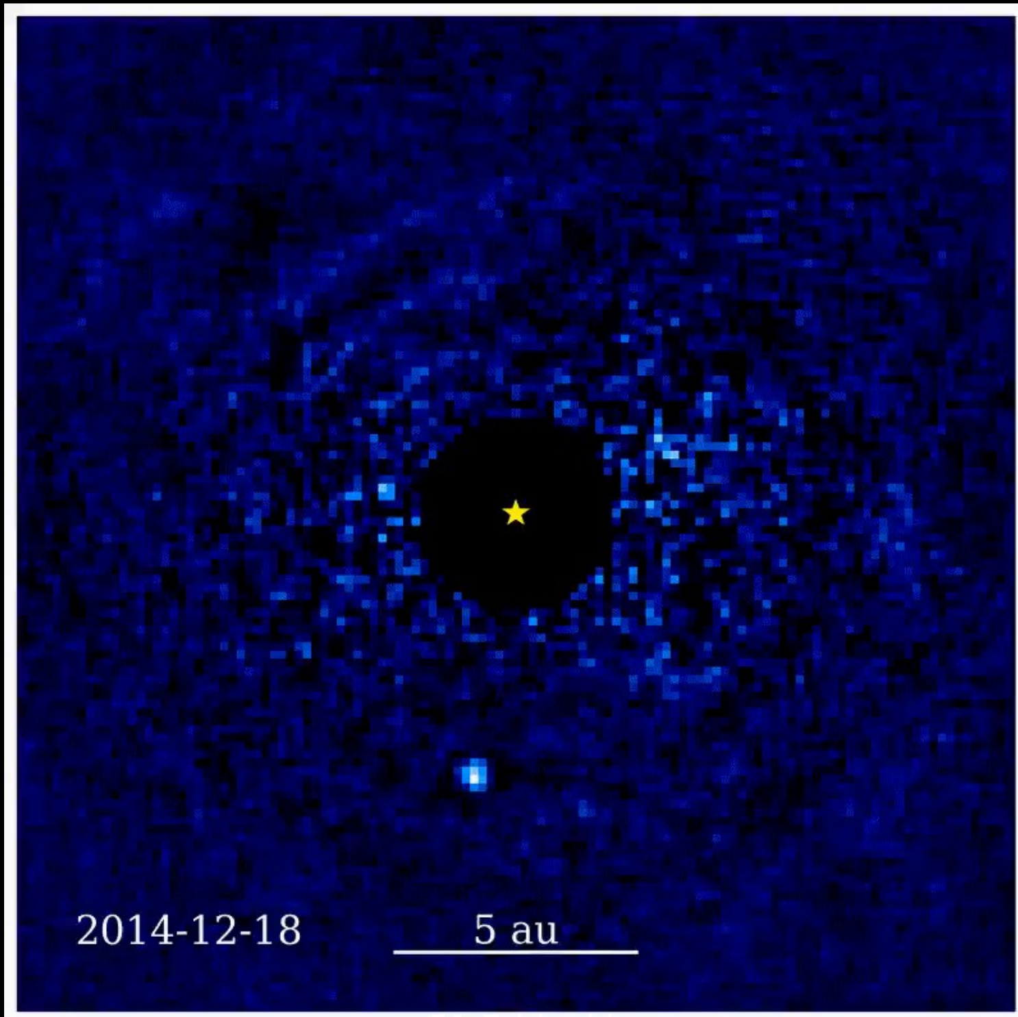
51 Eridani b
