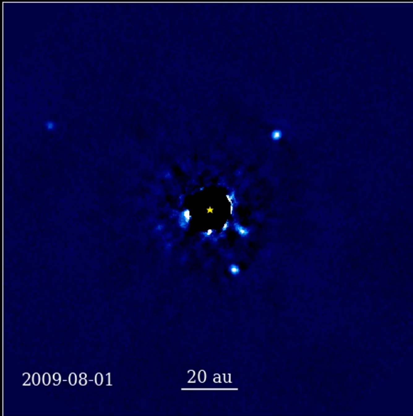
HR 8799 b,c,d,e
