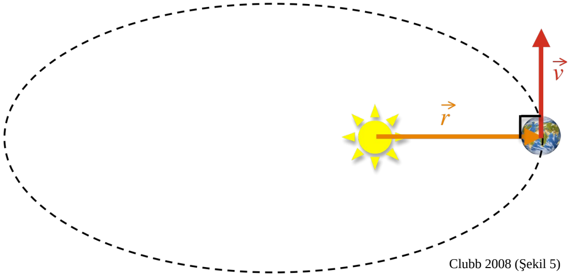
Şekil 3. Gezegenin yörünge hareketi boyunca konum vektörü r ile onun zamana göre türevi olan hız vektörü v , her zaman birbirine diktir.
