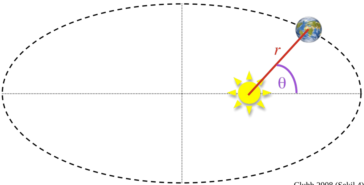
Şekil 2. Gerçek anomalî ( \theta ). Gezegenin konumu Dünya, yıldızın konumu Güneş görseli ile verilmiştir.
